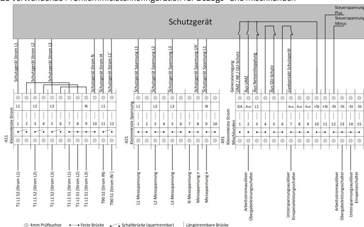
Abbildung 1, Prüfklemmleiste für Bezugs- und Mischkunden
