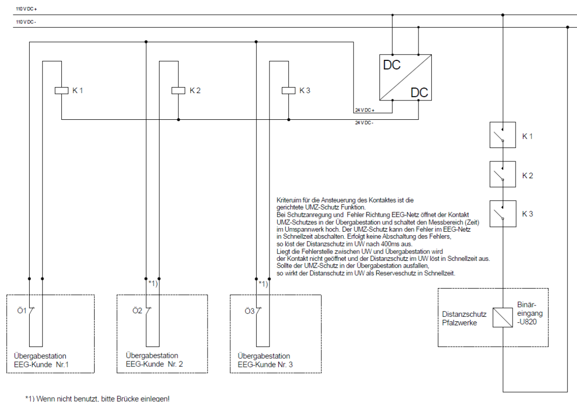
Abbildung 3, Rückwertige Verriegelung einer Erzeugungsanlage bei einem UW-Anschluss
