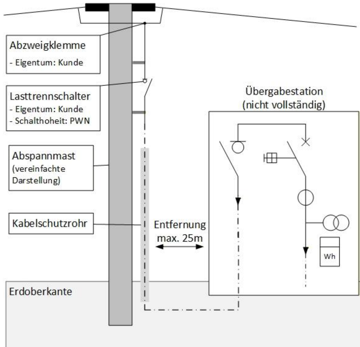
Abbildung 4, Beispiel für einen Freileitungsmastanschluss im Stich einer Übergabestation von einer EZA
