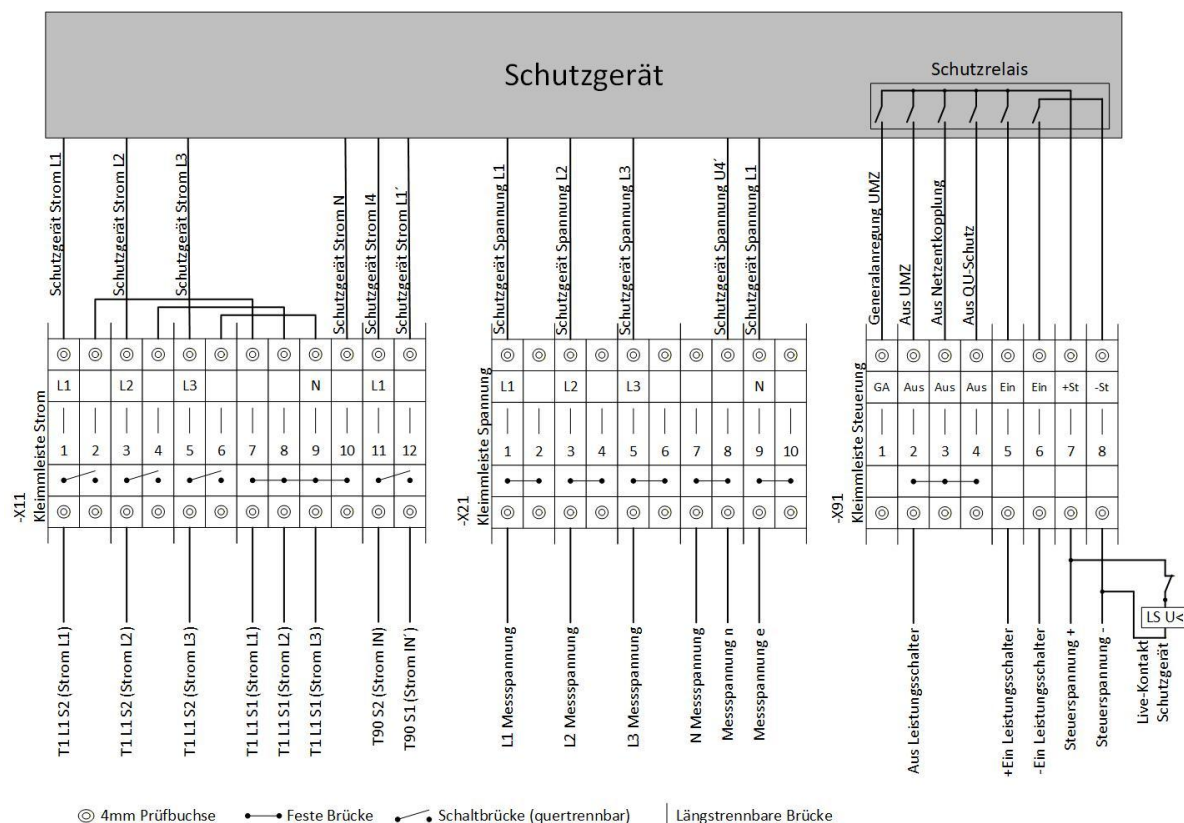
Abbildung 2, Prüfklemmleiste für Erzeugungsanlagen
