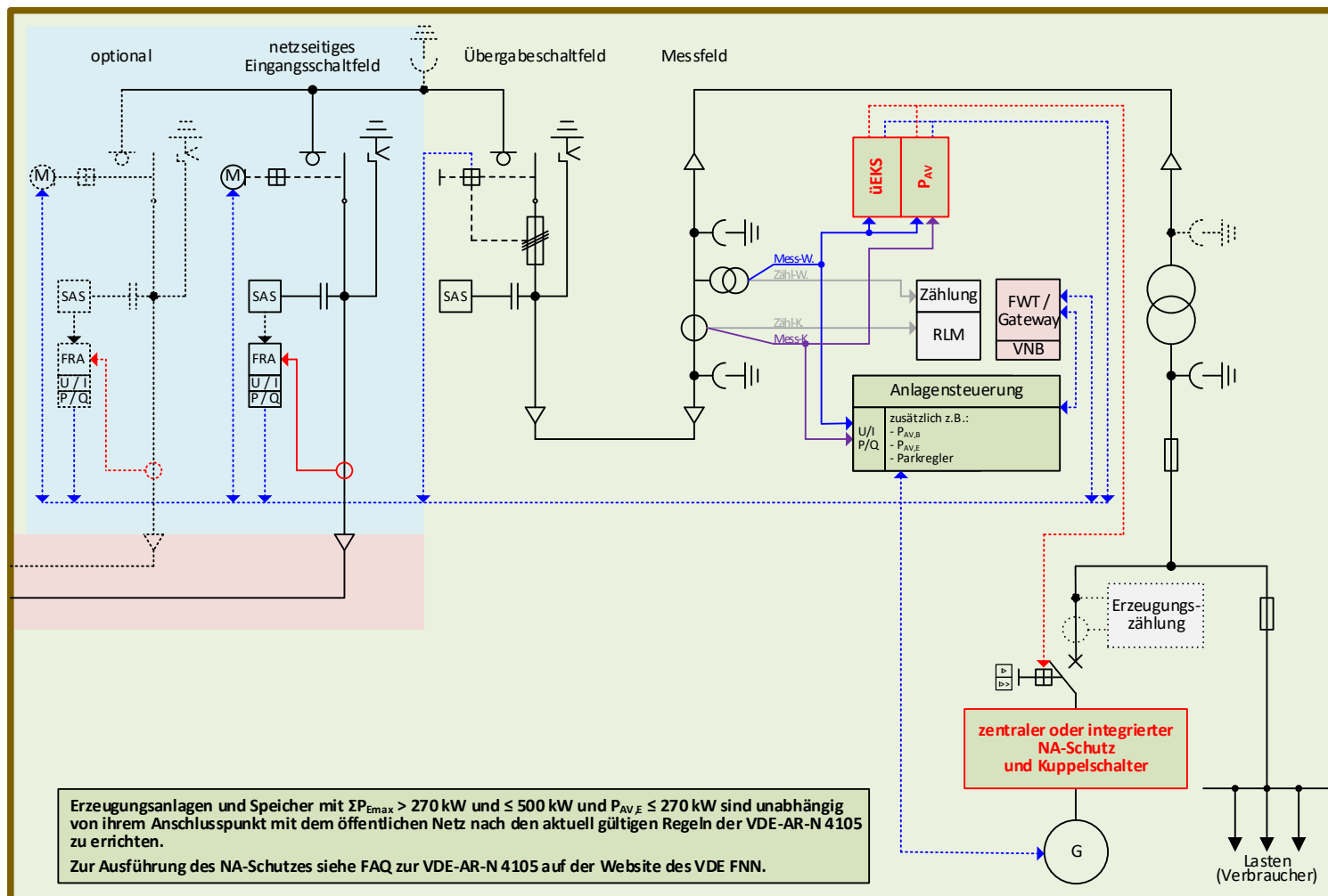
Bild D4b (K)K-TM und \Sigma P_{E_{max}} \leq 500 \text{ kW} und P_{AV,E} \leq 270 \text{ kW} :
